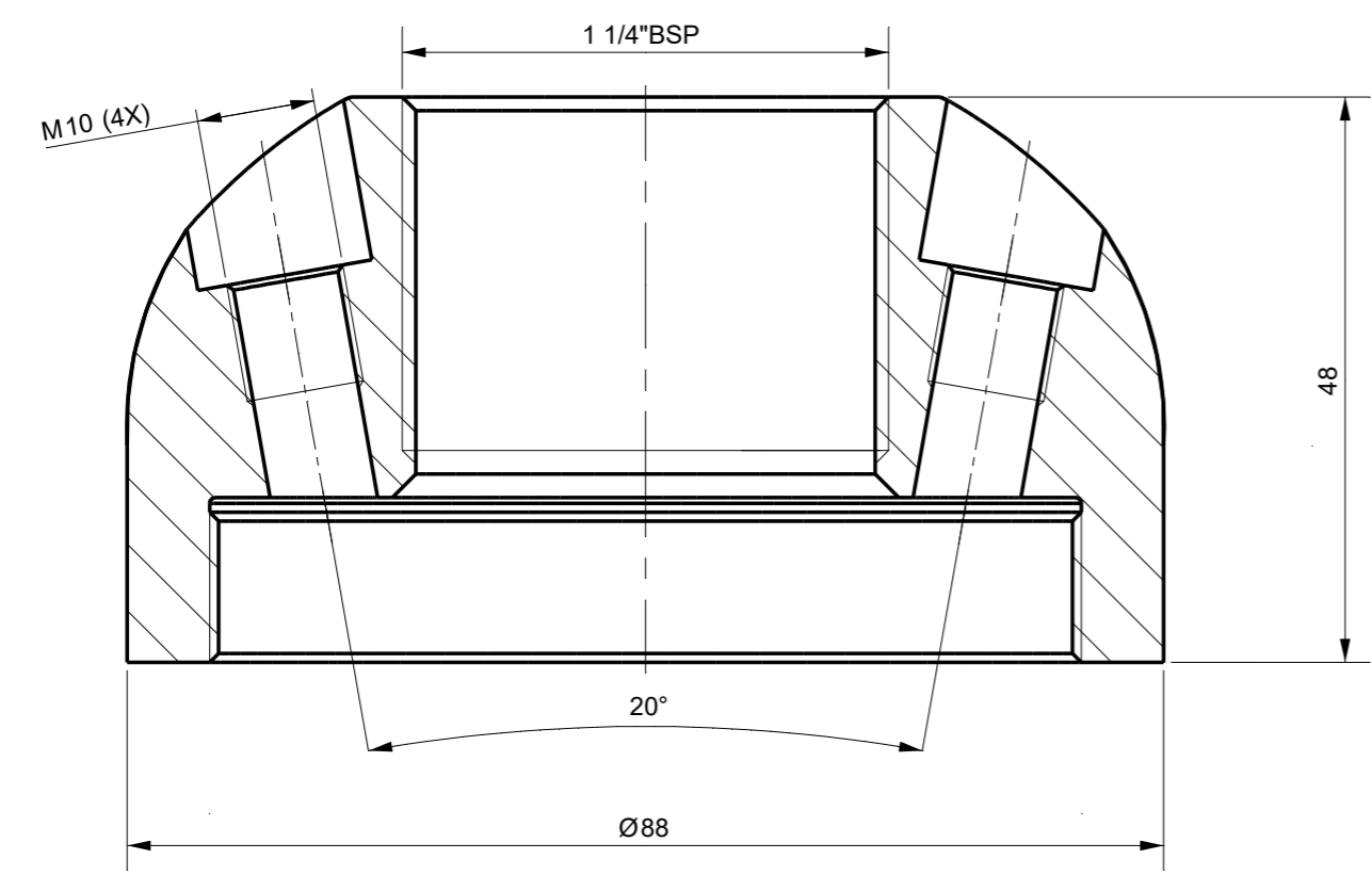
Section A-A
