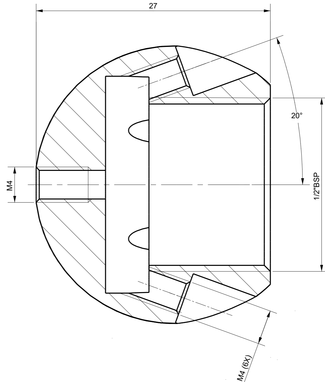
Section A-A
