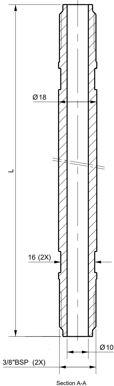
Section A-A
