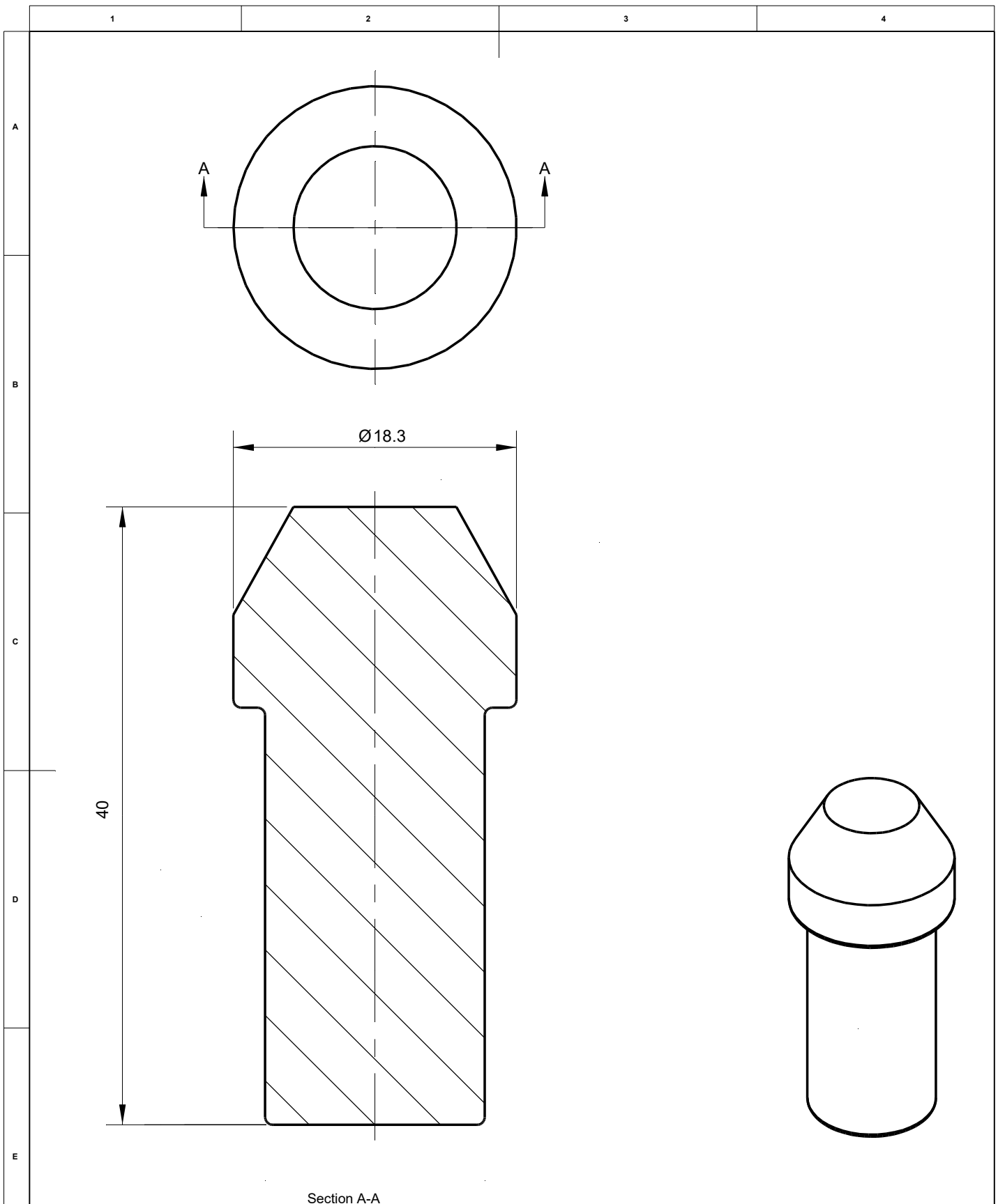
Section A-A
