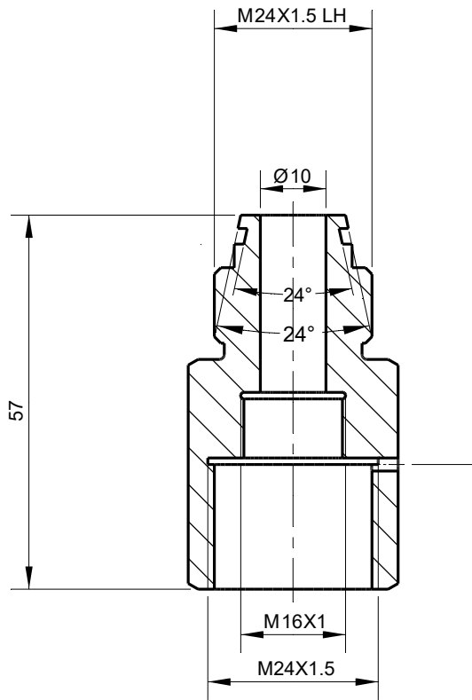
Section A-A
