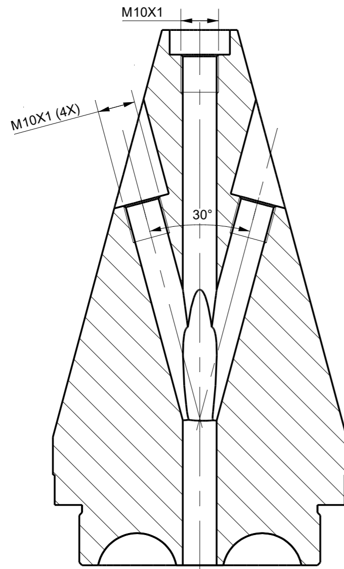
Section A-A
