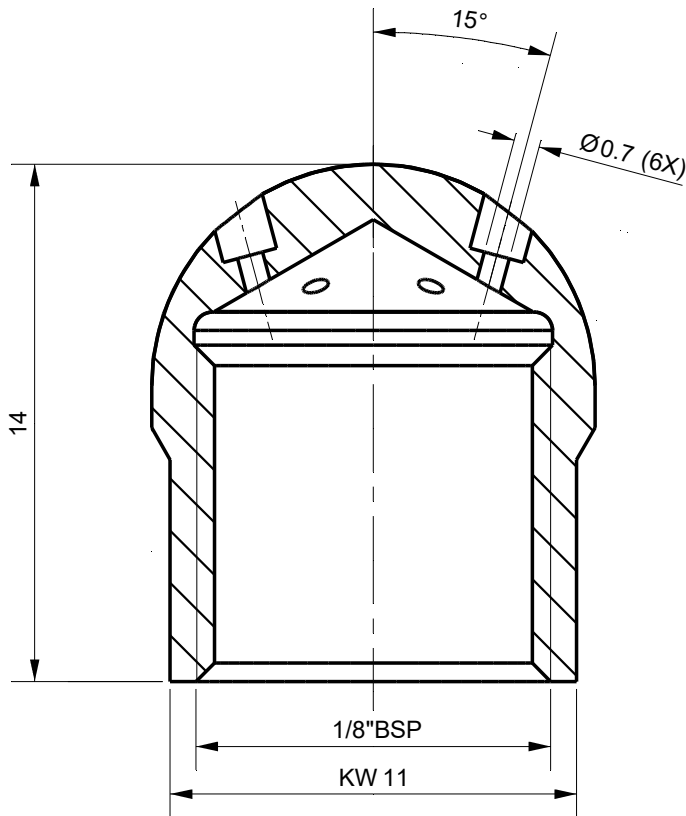
Section A-A
